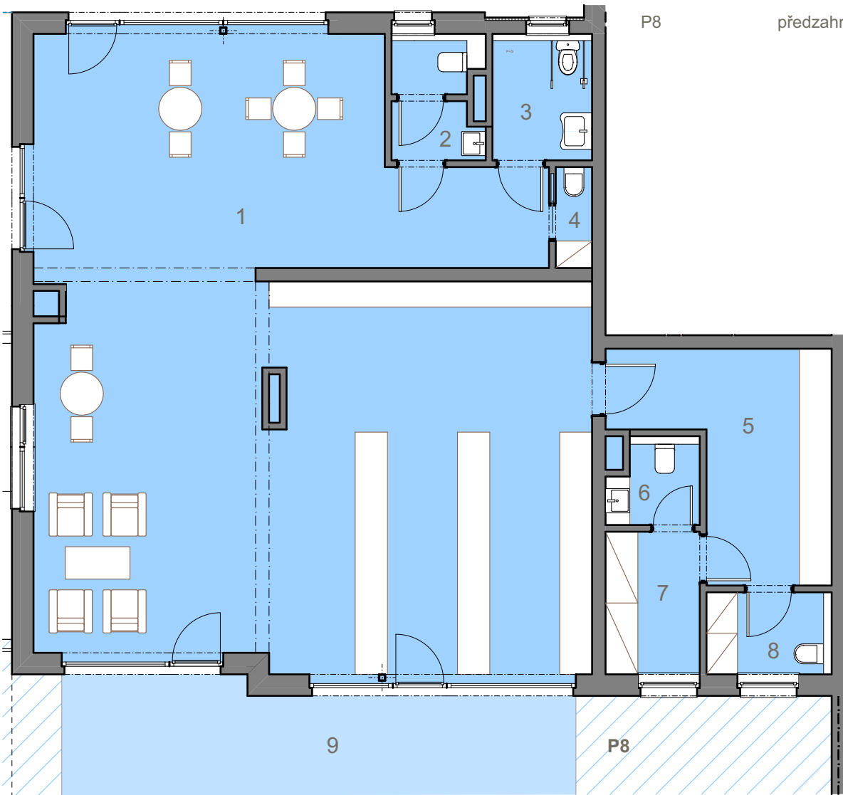
umístění jednotky v rámci podlaží a bytového domu
