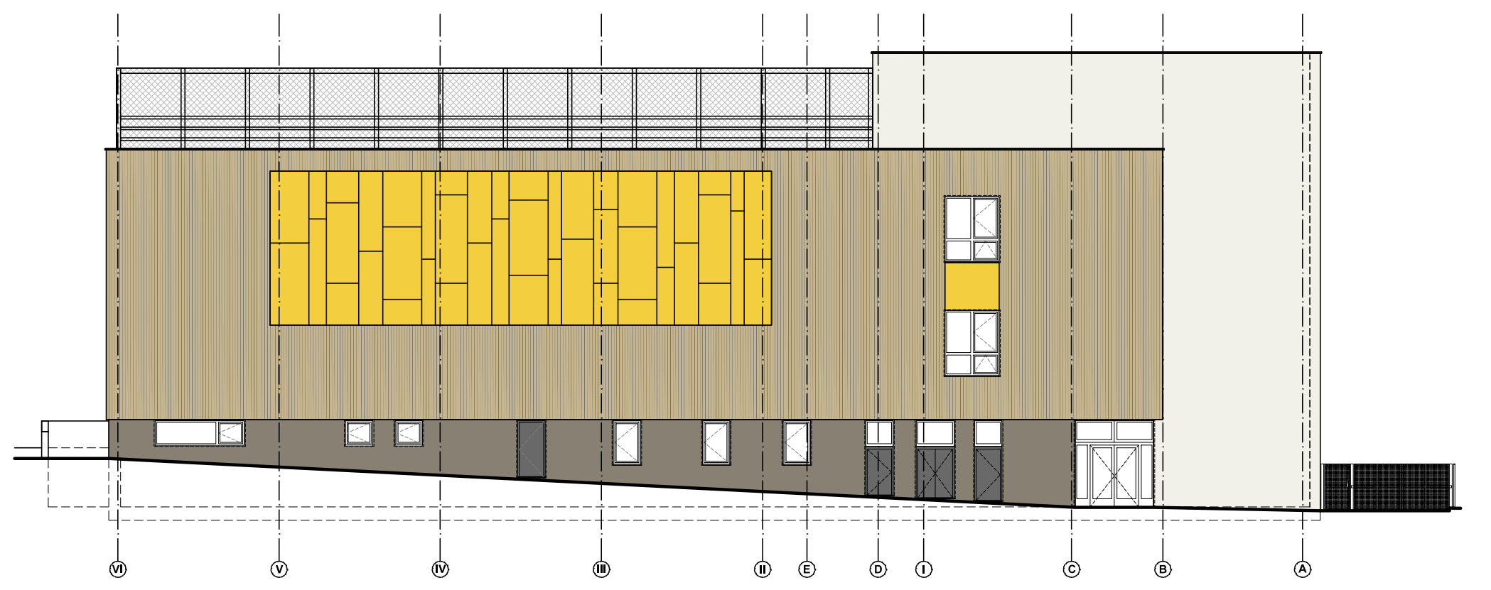
POHLED VÝCHODNÍ
